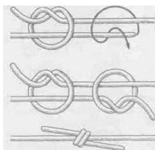
Брам-шкотовый узел
