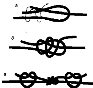
Брам-шкотовый узел
